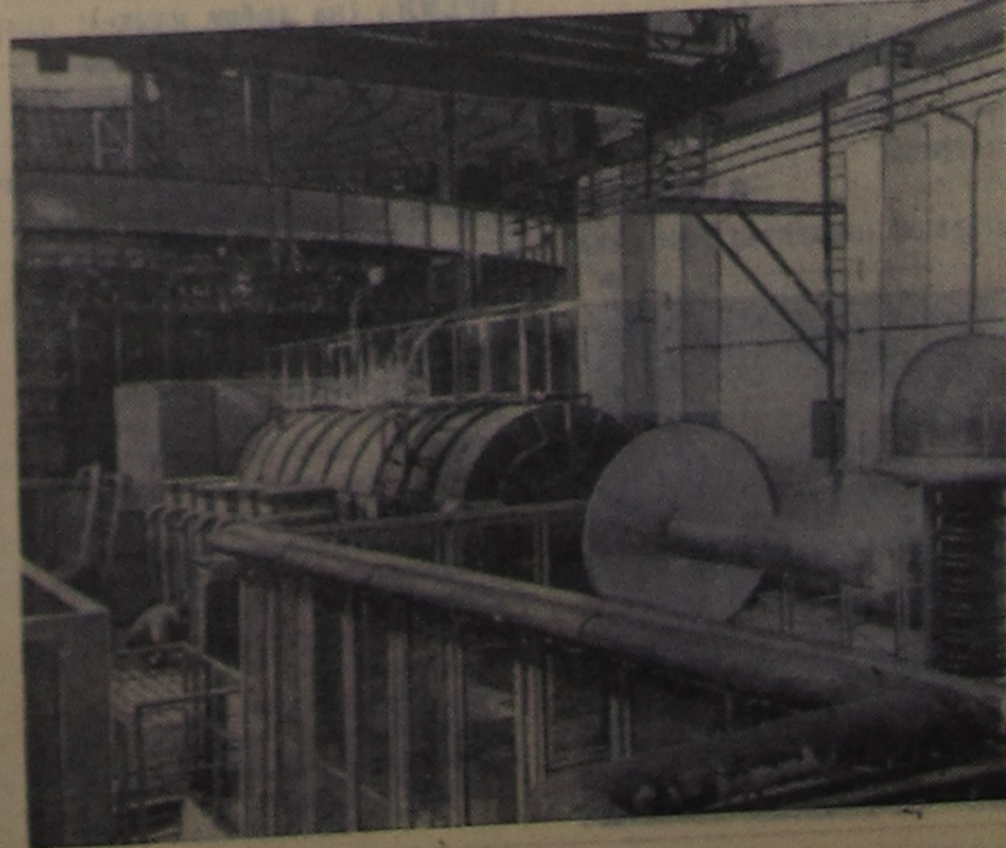
В Лаборатории высоких энергий. Форинжектор. Фото В. Шустина.
