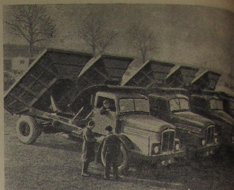
ГЕРМАНСКАЯ ДЕМОКРАТИЧЕСКАЯ РЕСПУБЛИКА. На Лейпцигской международной весенней ярмарке народное предприятие «Специальфаршейверк» в Берлине представило наряду с другими экспонатами самосвалы с обогреваемым снизу кузовом, предназначенные для транспортировки грузов в зимнее время. Полезная грузоподъемность машин — 7 тонн. Фото Центральбиля.
