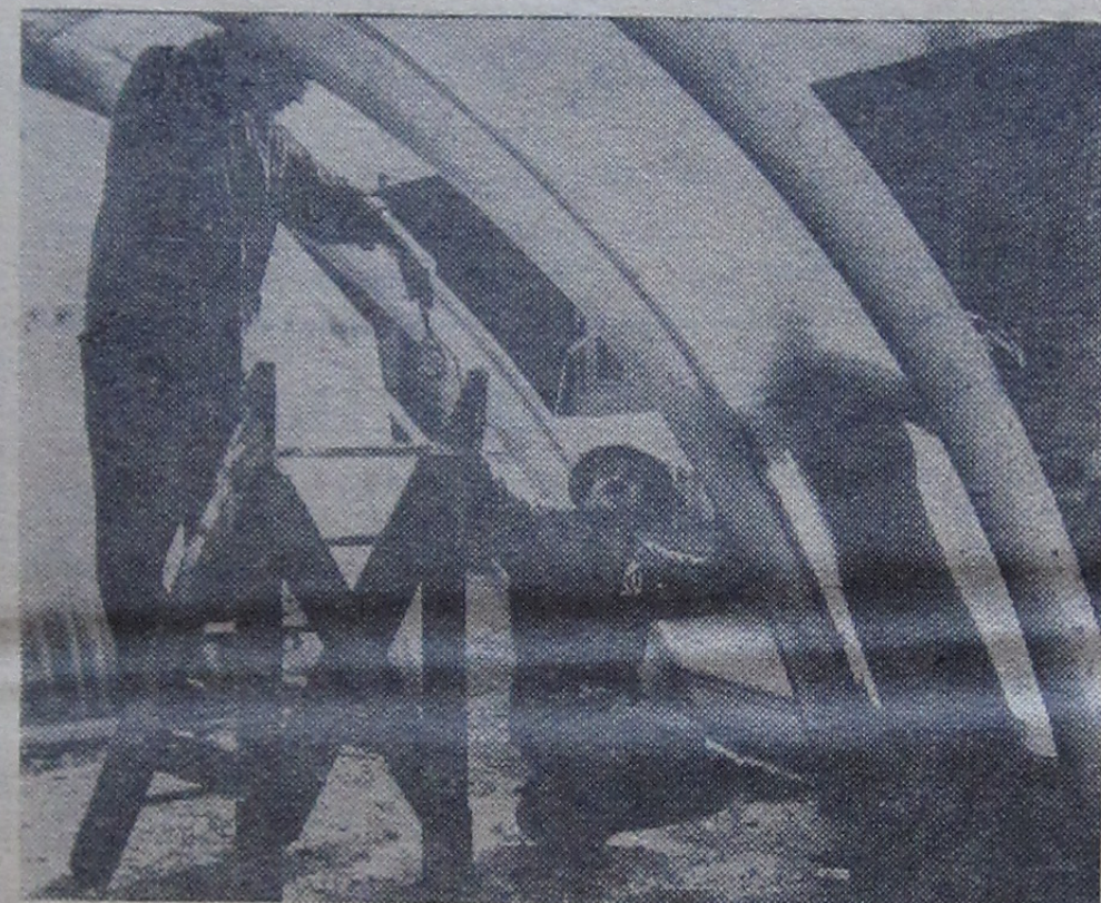
ЧЕХОСЛОВАЦКАЯ СОЦИАЛИСТИЧЕСКАЯ РЕСПУБЛИКА. Коллектив работников научно-исследовательского института строительной техники в Праге изучает возможности использования пластмасс для нужд сельского хозяйства. На снимке: сборка экспериментальной теплицы из пластмассы. Теплица подобного рода легко переносится с места на место. Она создается системой труб, наполненных горячей водой. Фото И. Шароха.
