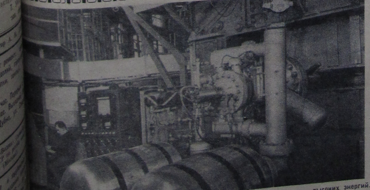
Эксперимент на метровой пузырьковой пропановой камере в Лаборатории высоких энергий. На фото — старший научный сотрудник Лаборатории ядерных проблем В. Б. Флягин.
