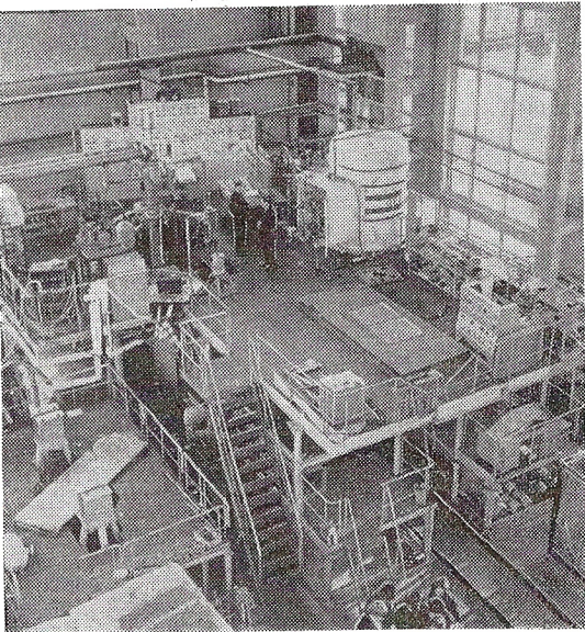
На снимке: установка с 2-метровой водородной камерой ОИЯИ во время третьего водородного пуска.
