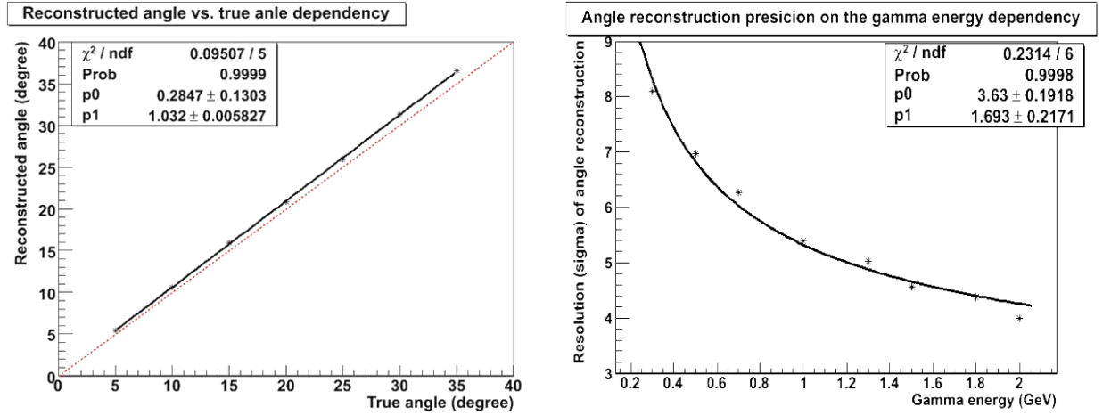
Рисунок 7 - Линейность восстановления направления \gamma -квантов (слева) и зависимость углового разрешения от энергии налетающих \gamma -квантов (справа). Пунктирная красная линия соответствует идеальному восстановлению. Результат (слева) получен обработкой Монте-Карло событий с энергией \gamma -кванта 1000 МэВ.
