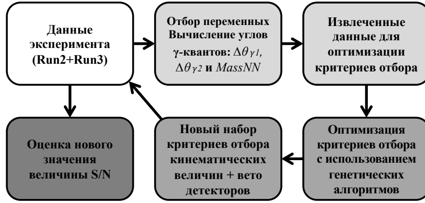
Рисунок 10 - Схема повторного анализа данных эксперимента E391a.
