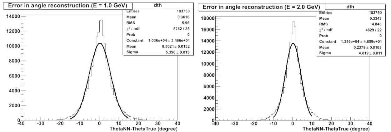
Рисунок 8 - Распределение абсолютной ошибки восстановления направления \gamma -квантов при энергиях 1 ГэВ (слева) и 2 ГэВ (справа). Угловое разрешение составило \sigma=5.4^\circ и \sigma=4.0^\circ соответственно.
