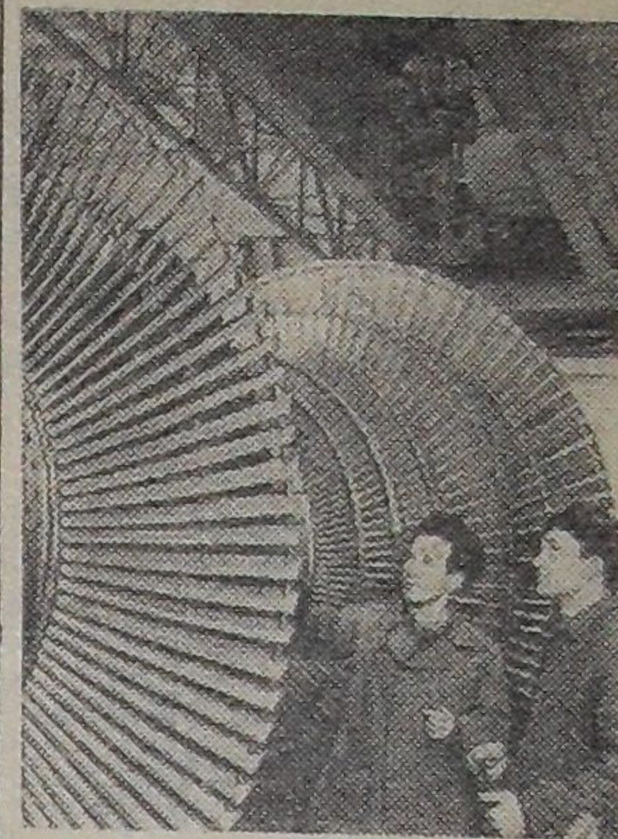
На снимке: слесари-монтажники В. И. ГРЕБНЕВ (слева) и С. Д. МАЛНОВ осматривают ротор паровой турбины перед установкой. Фото А. Грахова.
