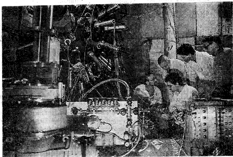
На снимке: установка ФАЗА для исследования ядерной мультифрагментации на пучке синхрофазотрона ОИЯИ. Участники коллаборации: профессор Х. Ойшлер, профессор Э. Норбек (США), Р. Барт, Ф. Липс (ФРГ), профессор В. А. Карнаухов.
