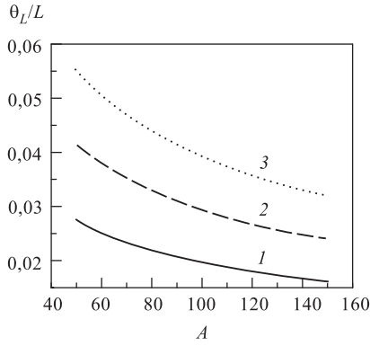
Рис. 3. Зависимость функции \theta_L/L от массового числа A : 1 — B = 4 кГц; 2 — B = 6 кГц; 3 — B = 8 кГц
