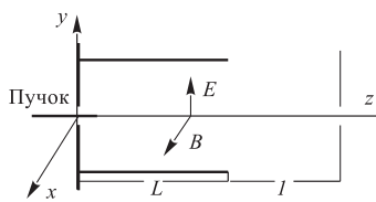
Рис. 2. Схема фильтра Вина, принятая в рассматриваемой модели
