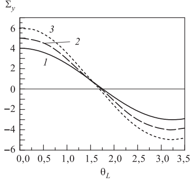
Рис. 5. Зависимость функции \Sigma_y от \theta_L : 1 — l/L = 3 ; 2 — l/L = 4 ; 3 — l/L = 5
