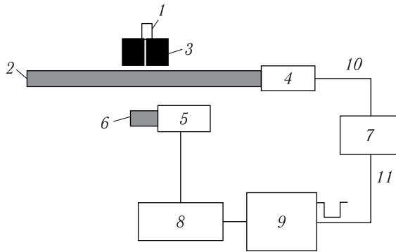
Рис. 15. Схема стэнда для проведения измерений с радиоактивным источником: 1 — бета-источник ^{106}\text{Ru} ; 2 — исследуемый образец; 3 — коллиматор; 4, 5 — SiPM; 6 — счетчик запуска; 7 — ЗЦП; 8 — усилитель; 9 — дискриминатор; 10 — измеряемый сигнал; 11 — сигнал разрешения
