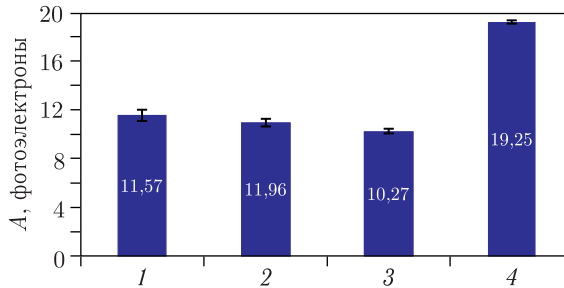
Рис. 37. Результаты измерения световыхода с квадратных тайлов, покрытых светоотражающим материалом разного типа: 1 — пленка Tyvek; 2 — пленка PolyTiO 2 ; 3 — белая краска на основе TiO 2 ; 4 — пленка ESR
