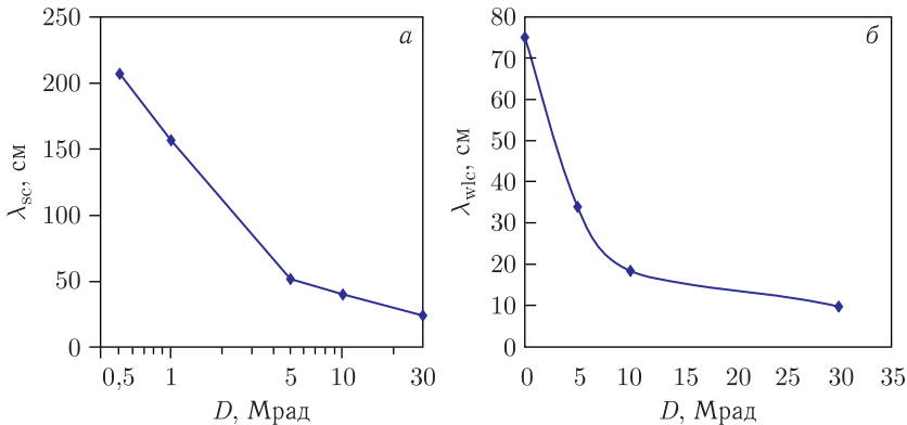
Рис. 8. Значения «измеренных» коэффициентов поглощения света в сцинтилляторе \lambda_{\text{sc}} (а) и в переизлучателе \lambda_{\text{wls}} (б) для каждой величины поглощенной дозы
