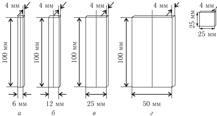
Рис. 5. Набор образцов секций для определения факторов, используемых в формуле (1)
