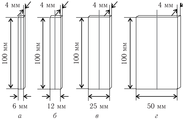
Рис. 2. Форма и размеры полос-секций и расположение переизлучателей в каждой секции
