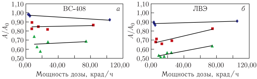
Рис. 29. Распределения световыхода ( A ) с облученных образцов BC-408 (а) и ЛВЭ (б), нормированные на световыход ( A_0 ) с необлученного образца, в зависимости от мощности дозы (ромбы — от 1,0 до 1,4 Мрад; квадраты — от 3,6 до 4,8 Мрад; треугольники — от 7,3 до 10 Мрад)
