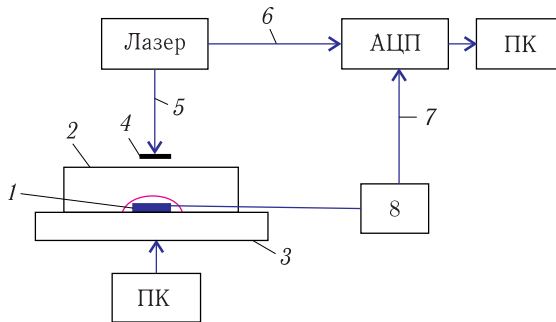
Рис. 40. Блок-схема стенда по измерению световыхода с тайла: 1 — SiPM; 2 — образец-тайл с лункой; 3 — движущийся стол; 4 — фильтр света лазера; 5 — оптоволокно; 6 — сигнал запуска; 7 — измеряемый сигнал; 8 — усилитель
