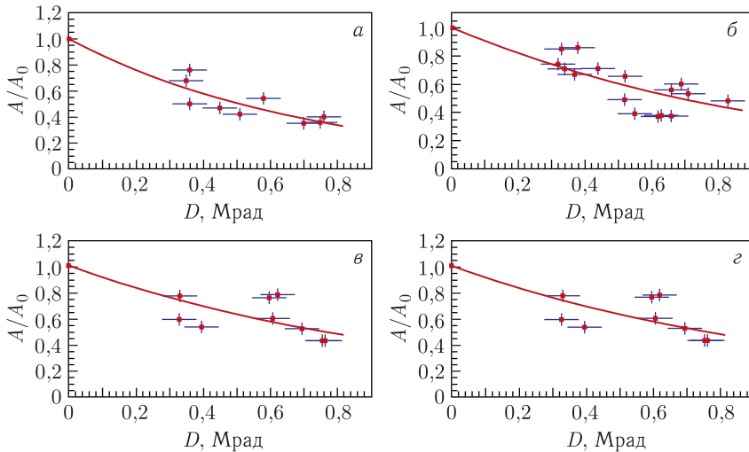
Рис. 49. Зависимости относительного световыхода от поглощенной дозы для тайлов, обернутых ESR, для четырех типов сцинтилляторов: а) SC-301; б) UPS-923A; в) BC-408; г) SC-307
