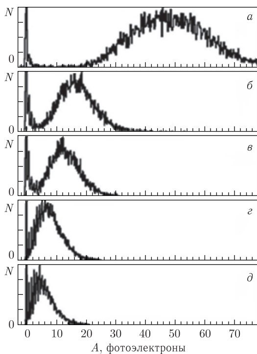
Рис. 16. Распределения амплитуд сигналов с образцов (BC-408), облученных до 25 Mrad при следующих значениях мощности дозы: а) необлучен; б) 0,6 Mrad/ч; в) 0,2 Mrad/ч; г) 0,04 Mrad/ч; д) 0,02 Mrad/ч
