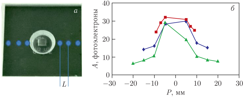
Рис. 43. Сканируемый тайл (вид сверху) (а) и результаты по сканированию (с шагом L ) лазером поверхности тайлов (б): ромбы — 30 \times 30 мм; квадраты — 20 \times 20 мм; треугольники — 40 \times 40 мм
