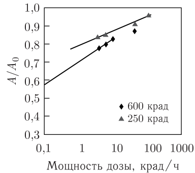
Рис. 13. Зависимости относительного световыхода от мощности дозы для облученных образцов сцинтиллятора SCSN-81. Измерения проведены спустя 7 сут после облучения (отношение сигналов A с облученных образцов к сигналу A_0 с необлученного образца)
