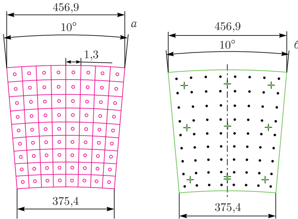
Рис. 53. Сцинтиляционная пластина с канавками и лунками (а) и печатная плата для размещения фотодетекторов и электроники считывания сигналов (б)
