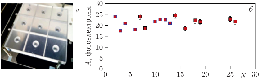
Рис. 56. а) Вид на моноблок тайлов, выделенных в пластине сцинтиллятора UPS-923A; б) зависимость световыхода от номера тайла в исследуемых моноблоках
