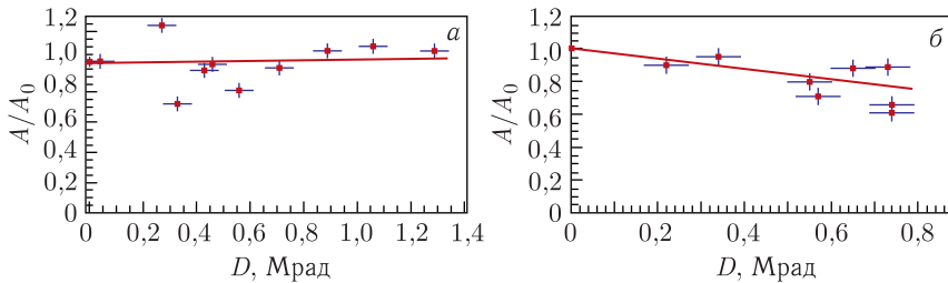
Рис. 50. Зависимости относительного световыхода от поглощенной дозы. Тайлы изготовлены из сцинтиллятора EJ-260, часть из которых обернута материалом Тувек (а), а часть — ESR (б)
