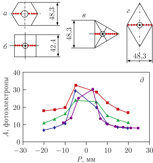
Рис. 44. Формы и площади поверхностей тайлов: а) шестиугольник, 1798 мм 2 ; б) квадрат, 1800 мм 2 ; в) треугольник, 1167 мм 2 ; з) ромб, 2020 мм 2 ). д) Зависимости световыхода от положения пятна лазера на поверхности для каждой формы тайла: ромбы — квадрат; квадраты — шестиугольник; треугольники — ромб; кружки — треугольник
