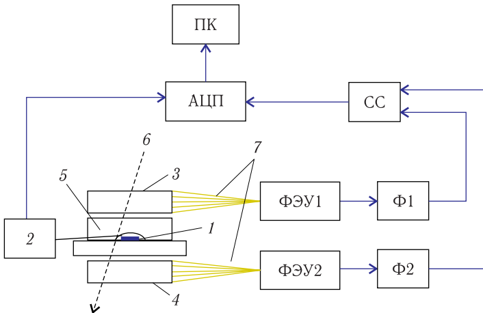
Рис. 35. Блок-схема стенда для измерения световыхода с образцов для исследования световыхода с использованием космических мюонов: 1 — SiPM на подложке; 2 — усилитель; 3, 4 — сцинтилляторы для выделения космического мюона; 5 — образец с лункой для размещения SiPM; 6 — трек космического мюона; 7 — оптоволоконна; Ф1, Ф2 — формирователи сигналов с ФЭУ1 и ФЭУ2; СС — схема совпадений сигнала разрешения для АЦП
