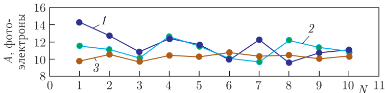
Рис. 39 (цветной в электронной версии). Повторяемость измерений световыхода с N образцов сцинтиллятора UPS-923A, отличающихся типом покрытия: синие кружки, 1 — пленка Tyvek; зеленые кружки, 2 — пленка PolyTiO 2 ; оранжевые кружки, 3 — белая краска на основе TiO 2
