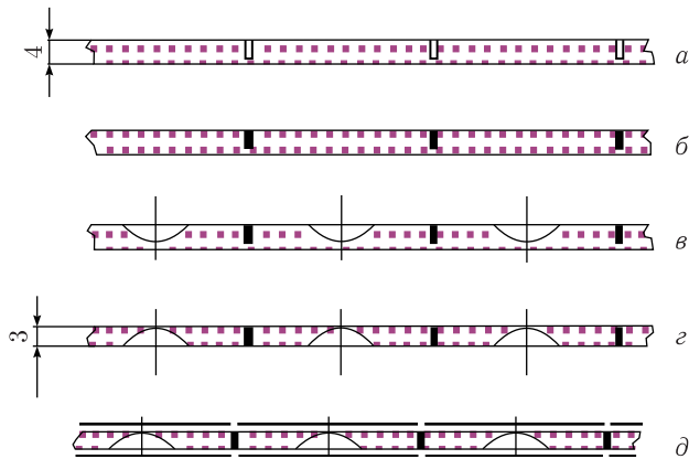
Рис. 54. Этапы формирования сцинтилляционных секций: а ) фрезерование канавок; б ) заполнение канавок непрозрачным составом; в ) фрезерование углублений; г ) удаление лишнего материала; д ) приклеивание зеркальной пленки сверху и снизу
