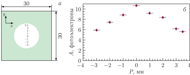
Рис. 52. а) Схематическое представление лунки в тайле и положение точек для измерения световыхода. б) Зависимость величины световыхода от положения SiPM относительно центра лунки
