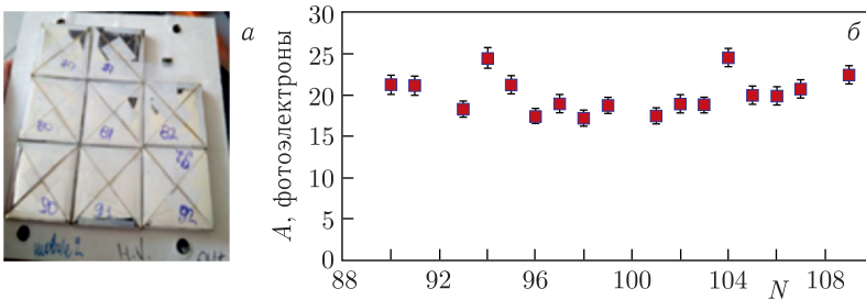
Рис. 57. а) Модуль, составленный из отдельных тайлов сцинтиллятора UPS-923A; б) зависимость световыхода от номера тайла в исследуемых модулях
