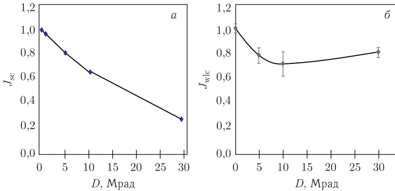
Рис. 9. Значения «измеренных» уровней деградации сцинтиллятора J_{sc} (а) и переизлучающего волокна J_{wlc} (б)
