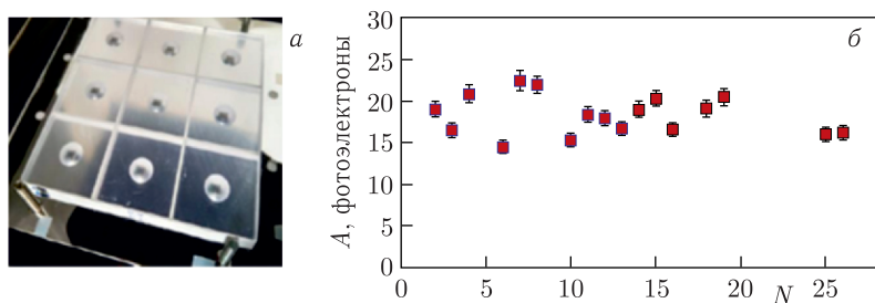
Рис. 58. а) Моноблок тайлов, выделенных в пластине сцинтиллятора BC-408; б) зависимость световыхода от номера тайла в исследуемых моноблоках
