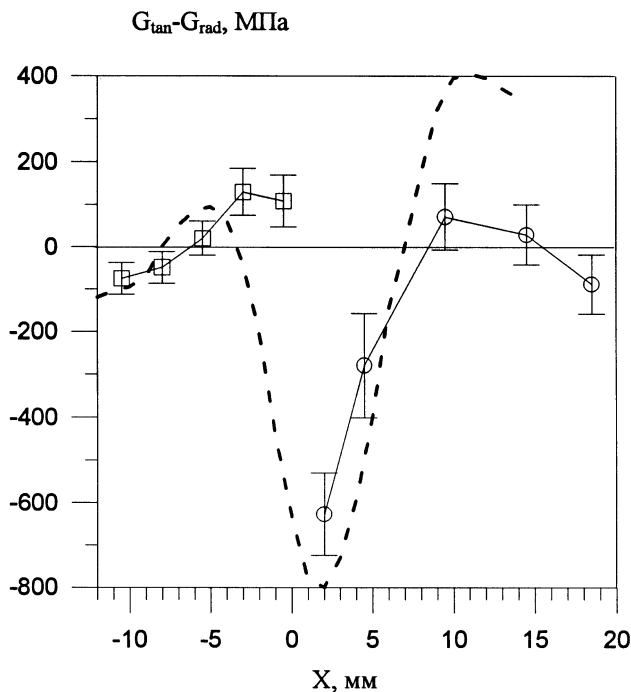
Рис. 11. Разность тангенциальной и радиальной компонент внутренних напряжений в трубе, показанной на рис. 10, измеренная в дифракционном эксперименте (□, ○) и полученная методом разрушающего контроля (пунктирная кривая) [41]
