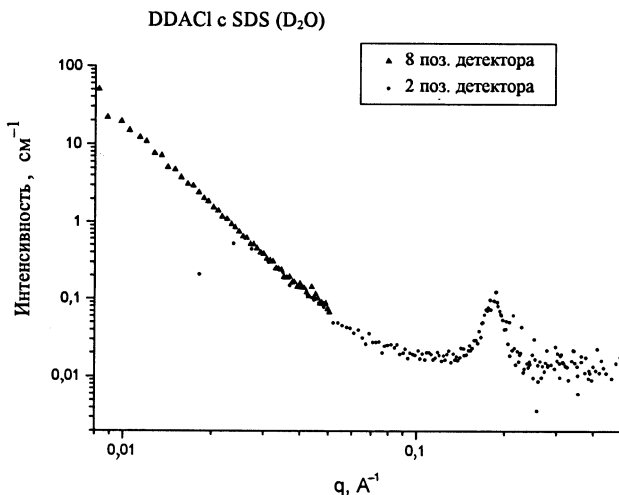
Рис. 3. Малоугловое рассеяние нейтронов в системе полимерный гель (диаллилдиметиламмонийхлорид)/ПАВ (додецилсульфат натрия)/D 2 O
