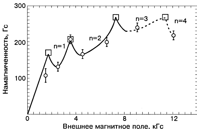
Рис. 9. Общая намагниченность YBa_2Cu_3O_7 пленки как функция внешнего магнитного поля. Прямая линия характеризует мейснеровское состояние. Сплошная линия, проходящая через экспериментальные точки (o), основана на расчетах [31], n означает количество рядов вихрей в пленке. Пустые квадратики ( \square ) обозначают величину внешнего магнитного поля, при котором имеют место переходы рядов вихрей.
