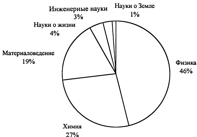
Рис. 16. Использование пучкового времени в различных науках по данным Европейской ассоциации по рассеянию нейтронов
