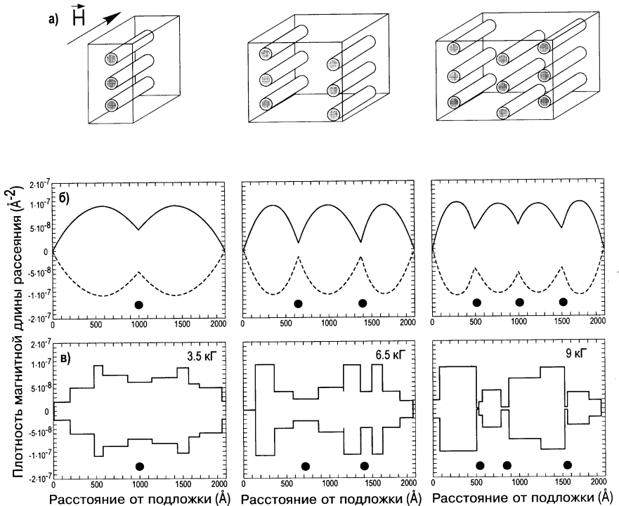
Рис. 8. Расположение рядов вихрей внутри сверхпроводящей тонкой пленки во внешнем магнитном поле \vec{H} . а) Схематическое изображение расположения от 1 до 3 рядов вихрей. б) Идеальный профиль плотности магнитной длины рассеяния (профиль намагниченности) на рядах вихрей, полученный с помощью рефлектометрии поляризованных нейтронов. Два спиновых состояния нейтрона во внешнем магнитном поле дают две плотности магнитной длины рассеяния и обозначены сплошной и пунктирной линиями. Ядерная плотность длины рассеяния не включена. в) Экспериментально полученная плотность магнитной длины рассеяния (профиль намагниченности) в представлении ступенчатой функции [30]. Данные были получены при температуре 4 К и охлаждении образца в нулевом поле
