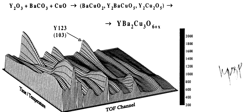
Рис. 4. Серия нейтронных дифракционных спектров, полученная в процессе синтеза высокотемпературного сверхпроводника YBa_2Cu_3O_x
