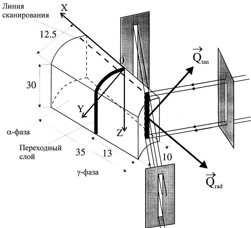
Рис. 10. Образец, вырезанный из трубы с наваренным ферритовым слоем. Показаны диафрагмы, ограничивавшие апертуры входного и рассеянного пучков [41]
