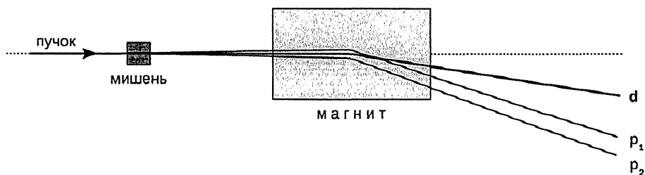
Рис. 7. Схема эксперимента с использованием одноплечевого спектрометра, обеспечивающая отбор событий с вылетом из мишени двух протонов с близкими импульсами в переднем направлении.
