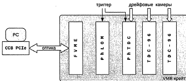
Рис. 9. Блок-схема системы сбора данных на установке. Сформированные сигналы с дрейфовых камер оцифровываются в модулях время-цифрового преобразования TDC-96 и PhTDC. Триггерный сигнал поступает на модули PhLOM и PhTDC. Интерфейсный FVME контроллер обеспечивает связь VME с удаленным компьютером по высокоскоростной оптической линии.
