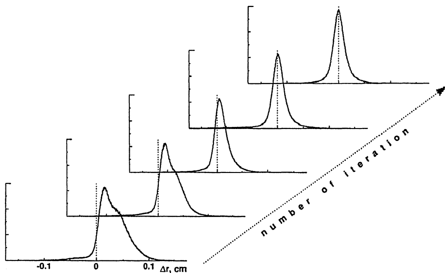
Рис. 10. Изменение распределения трекового остатка \Delta r в зависимости от номера итерации автокалибровки в дрейфовой камере.
