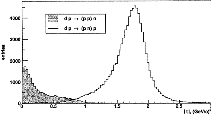
Рис. 2. Распределения событий реакции dp \rightarrow ppn по квадрату четырёхмерного переданного импульса |t| от протона-мишени к нейтрону.
