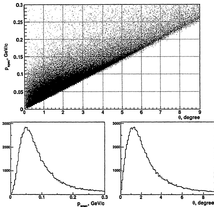
Рис. 4. Зависимость полярного угла вылета \theta нуклона-спектатора от его импульса p_{spec} из реакции развала дейтрона на протоне. Нижние распределения — проекции на соответствующие оси.
