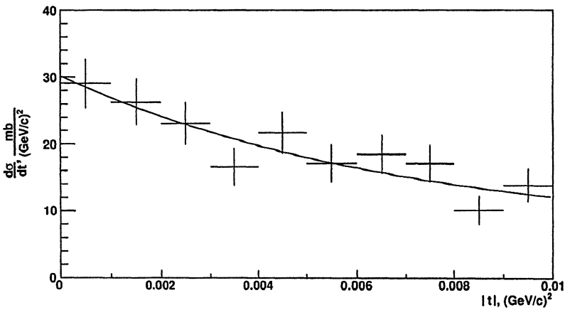
Рис. 5. Распределение дифференциального поперечного сечения реакции с обменом заряда dp \rightarrow (pp)n при малых значениях |t| .
