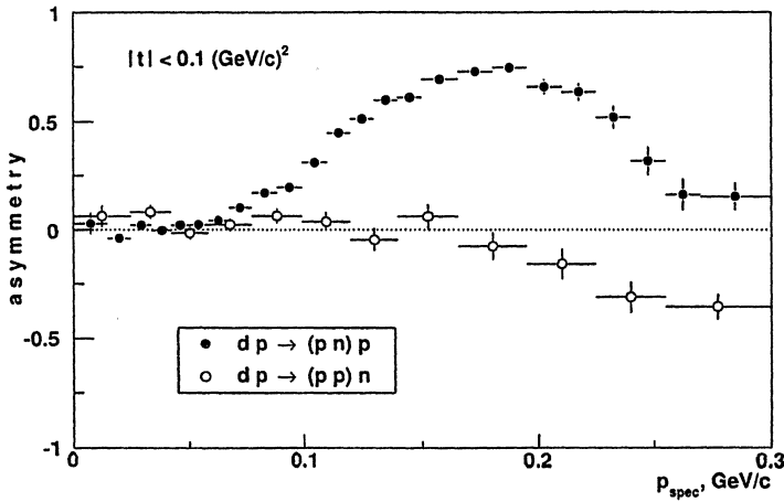
Рис. 3. Зависимость асимметрии по углу \alpha от импульса спектатора p_{\text{spec}} в системе покоя дейтрона.
