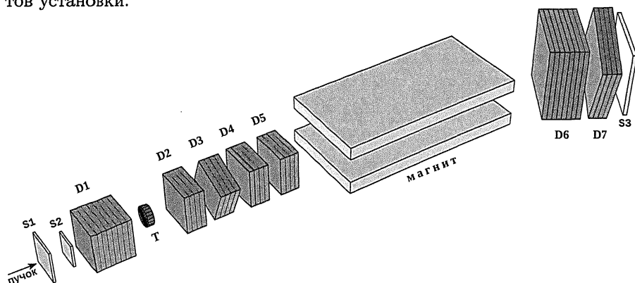
Рис. 8. Экспериментальная установка СТРЕЛА. D1–D5 — блоки «маленьких» дрейфовых камер с размером рабочей области 12.5 \times 12.5 \text{ см}^2 , D6–D7 — блоки «больших» камер с размером 25.0 \times 25.0 \text{ см}^2 , S1–S3 — сцинтилляционные счётчики, Т — мишень.
