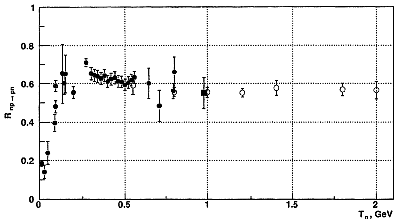
Рис. 6. Зависимость величины R_{np \rightarrow pn} от кинетической энергии нейтрона T_n . Сплошные кружки представляют значения, полученные в более ранних экспериментах, квадратик ( T_n = 0.98 ГэВ) — определённое нами значение, пустые кружки — недавно опубликованные результаты эксперимента Дельта-Сигма.
