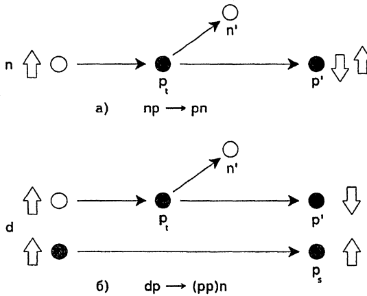
Рис. 1. Схематическое изображение а) элементарной реакции перезарядки нейтрона на протоне и б) перезарядки дейтрона на протоне-мишени.
