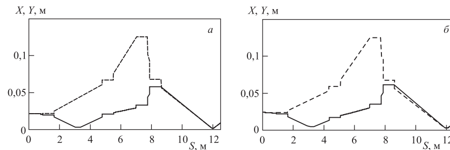
Рис. 3. Огибающие пучка X, Y вдоль канала для значений эмиттанса 25 \pi \text{ мм} \cdot \text{мрад} (a) и 50 \pi \text{ мм} \cdot \text{мрад} (б). Пунктиром показана огибающая Y
