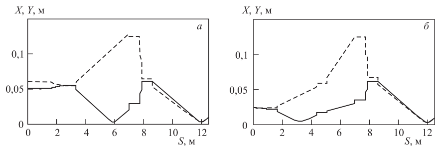
Рис. 8. Сравнение огибающих для конфигураций с различными начальными условиями — сечение в фокусе F3 0,1 \times 0,12 \text{ м} (а) и 0,04 \times 0,04 \text{ м} (б). Значение эмиттанса — 50 \pi \text{ мм} \cdot \text{мрад}
