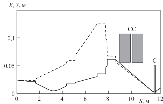
Рис. 2. Расположение сканирующей системы магнитов на пучке (CC). Область сканирования в фокусе пучка (C)
