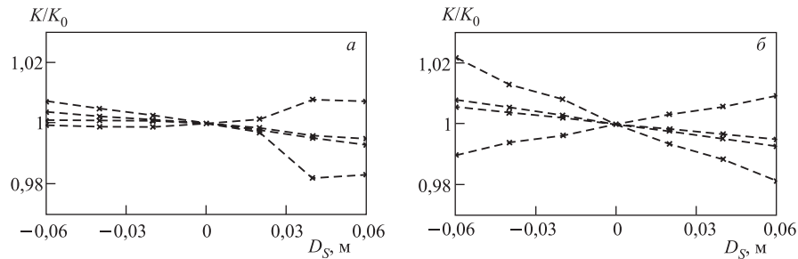
Рис. 5. Коррекция настройки линз, нормированная на значение в центральной точке. Значения эмиттанса — 25 \pi мм · мрад (а) и 50 \pi мм · мрад (б)
