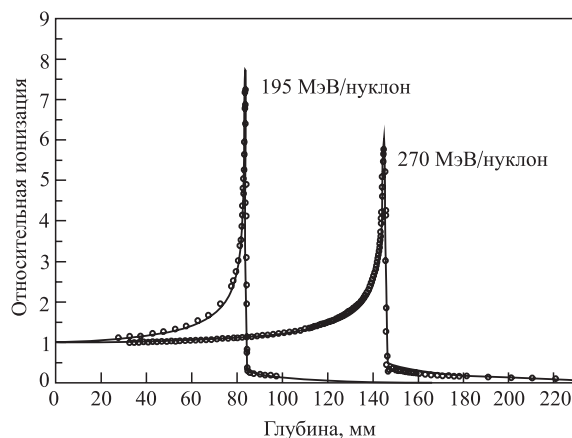
Рис. 6. Положение пика Брэгга при различных энергиях ионов углерода
