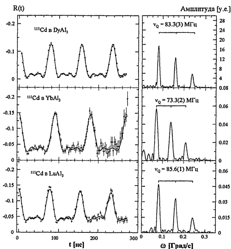
Рис.6. Спектры анизотропии для соединений \text{LnAl}_3 , (структурный тип \text{Cu}_3\text{Au} ).
