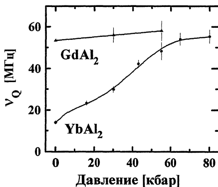
Рис.15. Зависимости квадрупольных частот от давления для ^{111}\text{Cd} в \text{YbAl}_2 и \text{GdAl}_2 .
