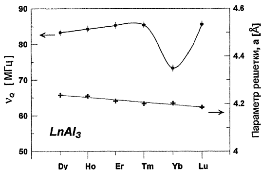
Рис. 8. Зависимости квадрупольной частоты и параметра решетки от Z лантаноида для соединений \text{LnAl}_3 , кристаллизованных в структурном типе \text{AuCu}_3 .
