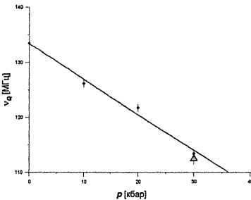
Рис.12. Зависимость квадрупольной частоты от давления для ^{111}\text{Cd} в Zn. Точки – данные из работы [9], треугольник наш результат.
