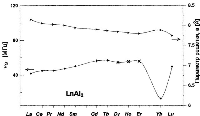
Рис.10. Зависимости квадрупольной частоты на ^{111}\text{In}(\text{Cd}) и параметра решетки для соединений \text{LnAl}_2 , от Z лантаноида.
