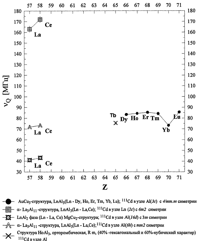
Рис.9. Зависимость квадрупольной частоты от Z лантаноида для соединений \text{LnAl}_3 .
