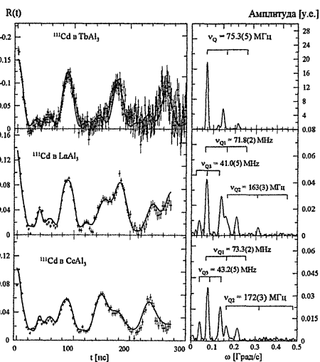
Рис.7. Спектры анизотропии для соединений \text{LaAl}_3 и \text{CeAl}_3 , (структурный тип \alpha\text{-La}_3\text{Al}_{11} ) и \text{TbAl}_3 , (структурный тип \text{HoAl}_3 ).
