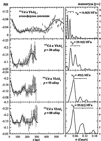
Рис.13. Образец \text{YbAl}_2
