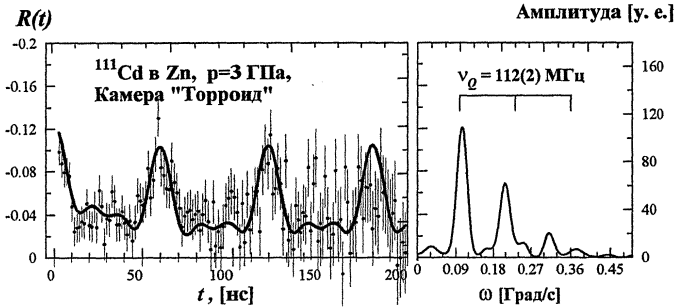
Рис.11. Спектр анизотропии ^{111}\text{Cd} в Zn измеренный при давлении 3 ГПа - камера типа „тороид”.
