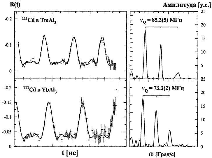
Рис.18. Спектры анизотропии угловой корреляции R(t) для ^{111}\text{Cd} в \text{TmAl}_3 и \text{YbAl}_3 , измеренные при нормальном давлении.
