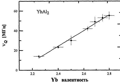
Рис.16. Зависимость квадрупольной частоты от валентности иона иттербия.
