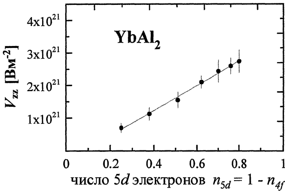
Рис.17. Зависимость ГЭП для ^{111}\text{Cd} в \text{YbAl}_2 от числа f электронов, перешедших в 5d зону ( 1 - n_{4f} = n_{5d} ).
