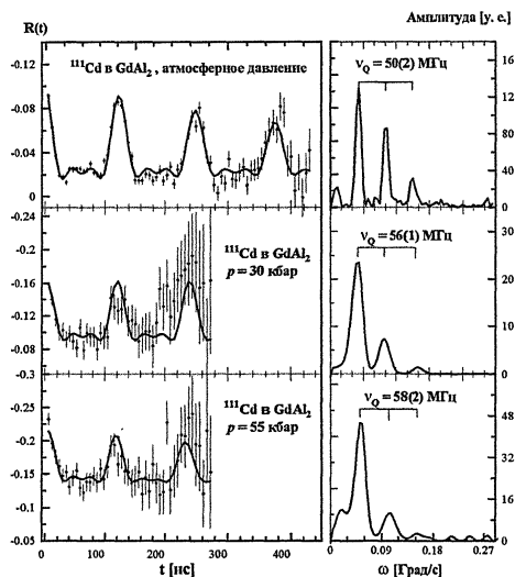
Рис.14. Образец \text{GdAl}_2
