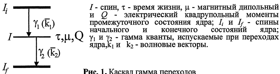
Рис. 1. Каскад гамма переходов
