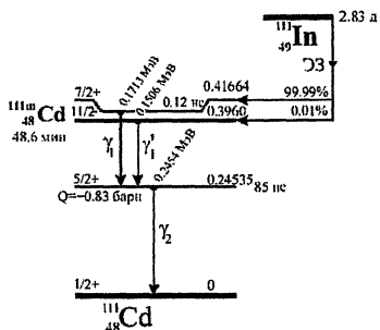
Рис.2. Схемы распада ^{111}\text{In} и ^{111\text{m}}\text{Cd} .
