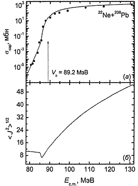
Рис.2. То же, что и на рис.1, только для реакции ^{22}\text{Ne} + ^{208}\text{Pb} .
