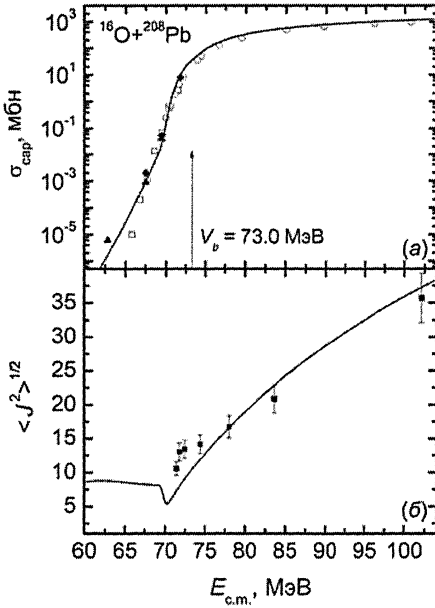
Рис. 1. Зависимости расчетных (сплошные кривые) сечений захвата (а) и среднеквадратичного углового момента системы после захвата (б) от E_{c.m.} для реакции ^{16}\text{O} + ^{208}\text{Pb} в сравнении с экспериментальными данными, показанными значками. Стрелкой обозначена величина кулоновского барьера.
