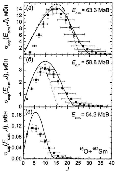
Рис. 6. Зависимости расчетных парциальных сечений захвата от J при фиксированных E_{\text{с.м.}} для реакции ^{16}\text{O} + ^{152}\text{Sm} . Расчеты с учетом статической деформации ядер изображены сплошными кривыми, без учета — штриховыми. Символами показаны экспериментальные данные.
