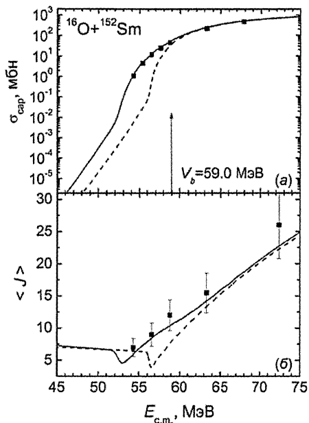
Рис. 5. Зависимости расчетных сечения захвата (а) и среднего углового момента системы после захвата (б) от E_{\text{с.м.}} для реакции ^{16}\text{O} + ^{152}\text{Sm} . Расчеты с учетом статической деформации ядер изображены сплошными кривыми, без учета — штриховыми. Символами показаны экспериментальные данные. Стрелкой обозначена величина кулоновского барьера в случае сферических ядер.
