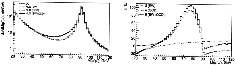
Рис. 1: Сравнение вкладов EW и QCD в поправки порядка NLO в распределении сечения по инвариантной массе лептонов в конечном состоянии для процесса Дрелла-Яна нейтрального тока pp \rightarrow \mu^+\mu^- .
