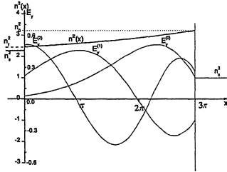
Рис. 1. Профиль показателя преломления (17) и собственные функции E_y^{(j)}(x) ( j = 0, 1, 2 ), d = 3\pi , \Delta = 0.181 .
