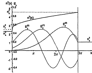
Рис. 2. Профиль показателя преломления с модификацией (19) ( \alpha = 1/3 ) и собственные функции E_y^{(j)} , d = 3\pi , \Delta = 0.4773 .
