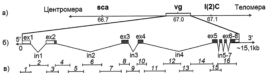
Рис. 1. ген vg , (а): генетическая карта района гена vestigial ; (б): схема экзонно-интронной структуры гена vestigial (15112п.н.); (г): положение ампликонов изучаемых субрайонов гена.
