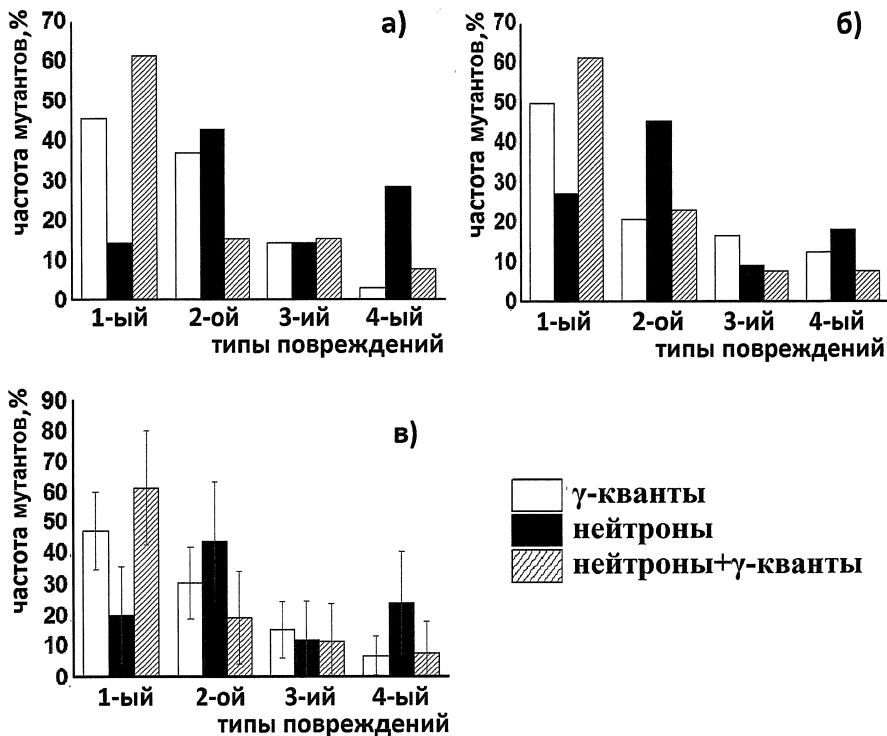
Рис. 2. Относительная частота мутантов \nu g с мутационными повреждениями 4 разных типов детектируемых методом ПЦР для изученных в работе видов излучений: а) мутанты «точковой» природы; б) мутанты абберационной природы; в) сумма двух выборок.
