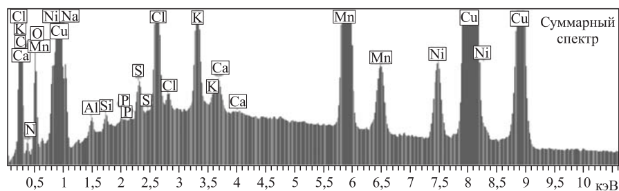
Рис. 26. Суммарный спектр РМЗА, соответствующий элементному составу при сканировании по полосе на рис. 25, а
