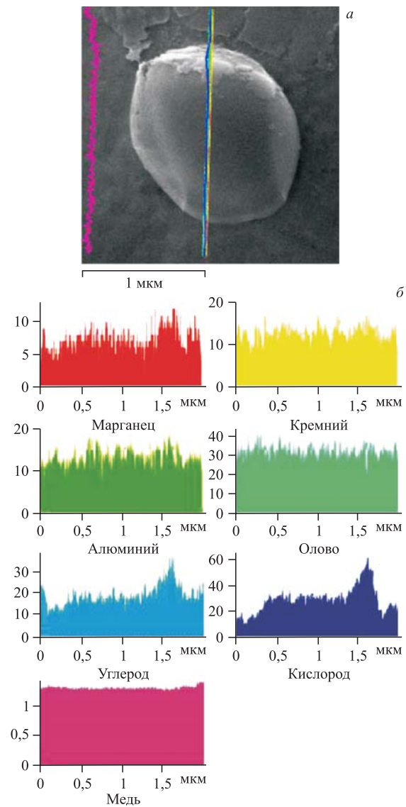
Рис. 29. СЭМ-изображение структуры с полосой сканирования РМЗА (а) и соответствующие распределения элементов (б)
