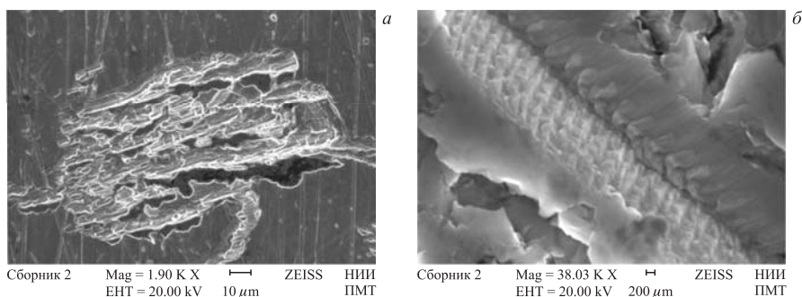
Рис. 34. СЭМ-изображения двух областей ЛС с меньшим \times 1,90 K (а) и большим \times 39,03 K (б) увеличениями
