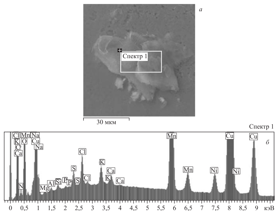
Рис. 27. СЭМ-изображение структуры ( a ) и ХСРИ, полученный с выделенной области (спектр 1) рис. 27, a ( б )
