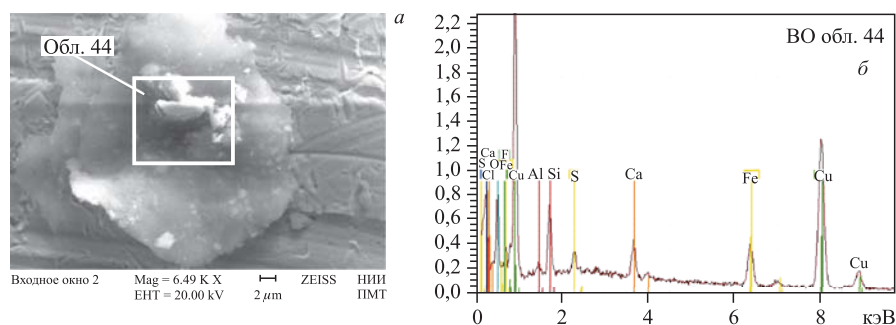
Рис. 10. СЭМ-изображения частицы на поверхности ВО с более мелкими структурами (а) и спектр РМЗА (б), измеренным в обл. 44
