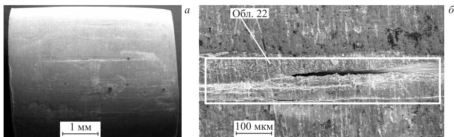
Рис. 12. СЭМ-изображения боковой поверхности Pd-стержня (а) и увеличенное изображение трещины на боковой поверхности и обл. 22 РМЗА (б)
