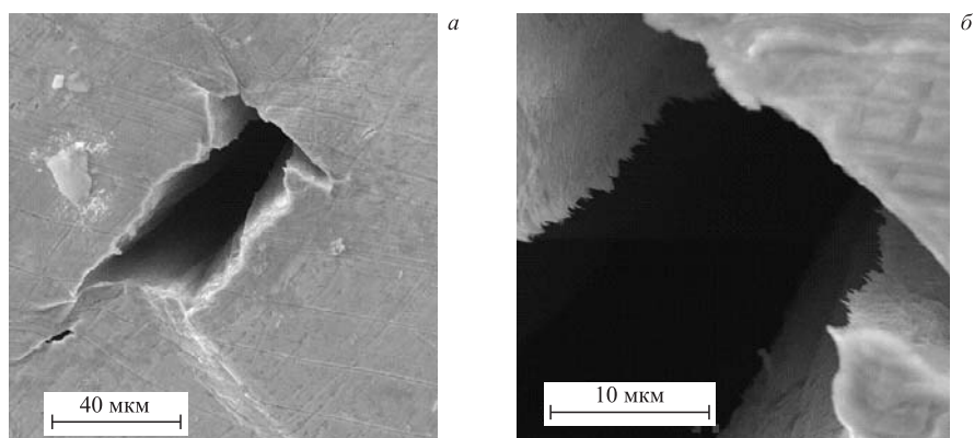
Рис. 20. СЭМ-изображения места разрыва поверхности Pd-стержня а ) с меньшим ( \times 2240 ) и б ) большим ( \times 10700 ) увеличением
