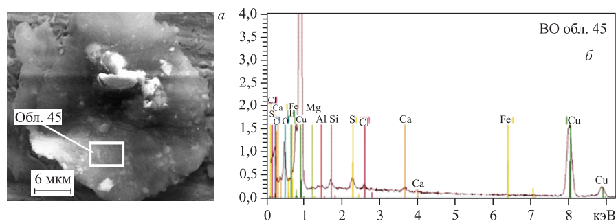
Рис. 11. СЭМ-изображение частицы на поверхности ВО (а) и спектр РМЗА в обл. 45 (б)
