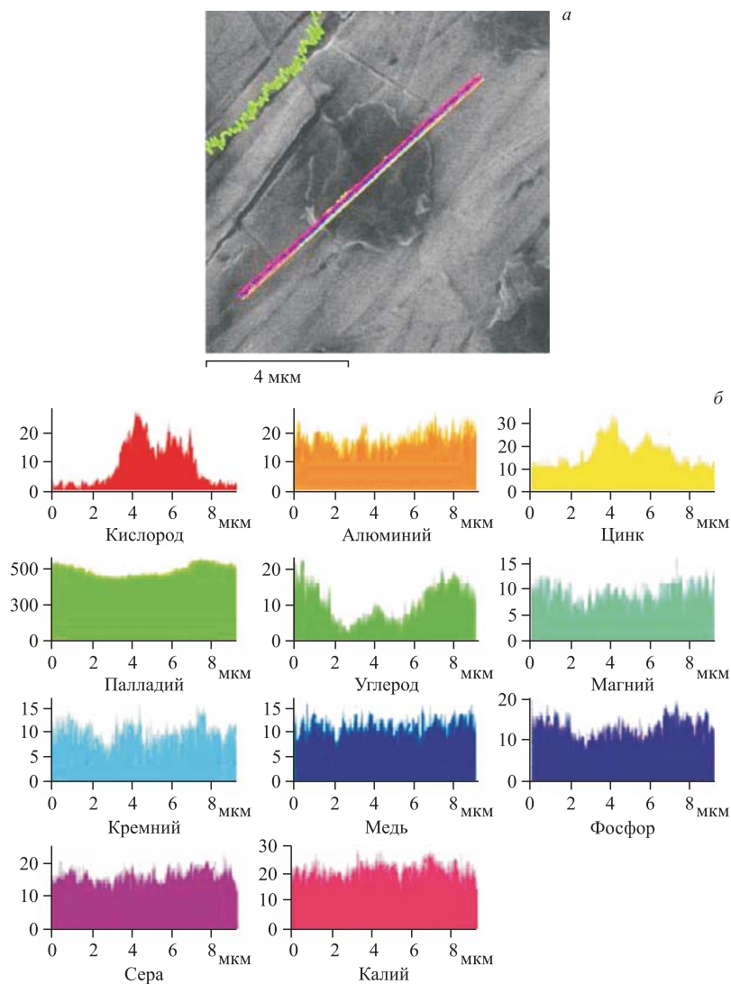
Рис. 22. СЭМ-изображение одиночного темного пятна, вдоль полосы на котором был сделан РМЗА ( а ), и спектры элементов ( б )
