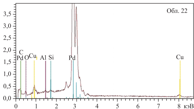
Рис. 13. Спектр РМЗА в обл. 22 на рис. 12, б
