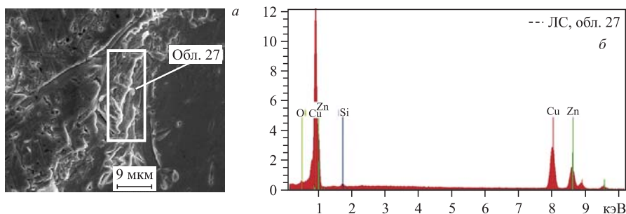
Рис. 31. СЭМ-изображение участка ЛС ( a ) и спектр РМЗА, измеренный в обл. 27 ( б )
