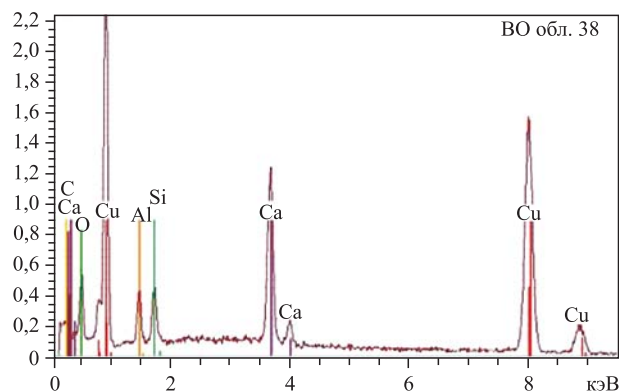
Рис. 3. Спектр РМЗА, измеренный на рис. 2, б в обл. 38 ВО
