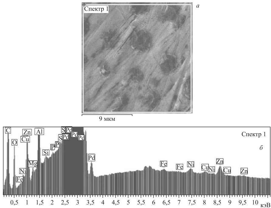
Рис. 21. СЭМ-изображение участка поверхности Pd-стержня в месте расположения темных пятен (а) и РМЗА-спектр со всей площади изображения (б)
