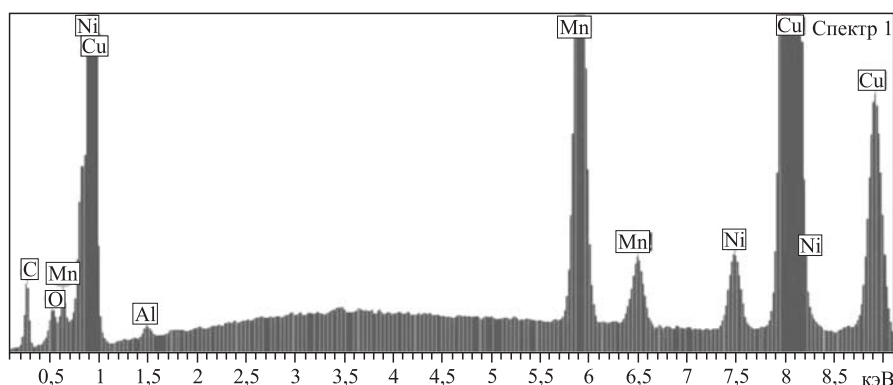
Рис. 23. Спектр РМЗА во внешне не измененной области манганиновой фольги
