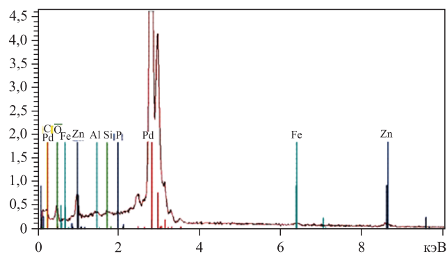
Рис. 18. Спектр РМЗА в обл. 26 на рис. 17, б
