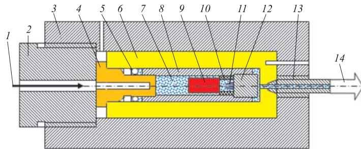
Рис. 1. Схематическое изображение ДНРС и ННРС: 1 — поток \gamma -квантов; 2 — уплотнение с входным отверстием; 3 — уплотнение для высокого давления в камере; 4 — \text{Cu}_{0,98}\text{Be}_{0,02} «входное окно»; 5 — уплотнение для высокого давления; 6 — \text{Cu}_{0,98}\text{Be}_{0,02} -стенки камеры высокого давления; 7 — дейтерий (ДНРС) или водород (ННРС); 8 — латунная втулка; 9 — Pd-стержень; 10 — разделительная фольга из марганца; 11 — синтезированный продукт реакции; 12 — латунный сборник; 13 — капилляр высокого давления; 14 — клапан и тензор-датчик давления
