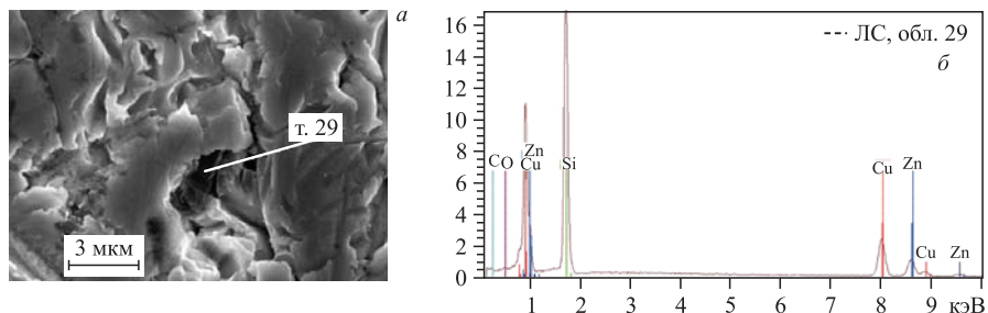
Рис. 33. СЭМ-изображение участка поверхности ЛС (а) и спектр РМЗА, проведенного в темной области в т. 29
