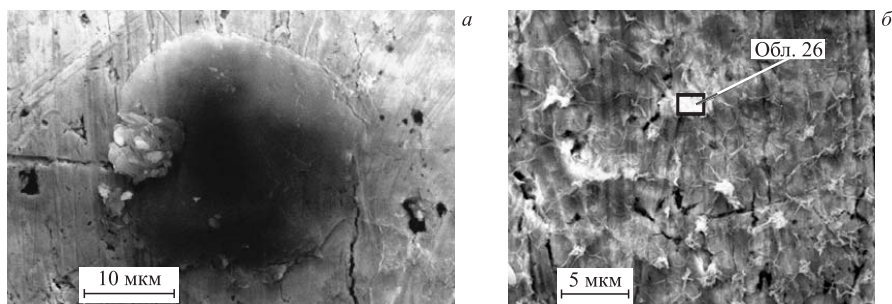
Рис. 17. СЭМ-изображения частицы (а) и участка поверхности Pd-стержня с мелкими частицами и РМЗА, проведенным в обл. 26 (б)
