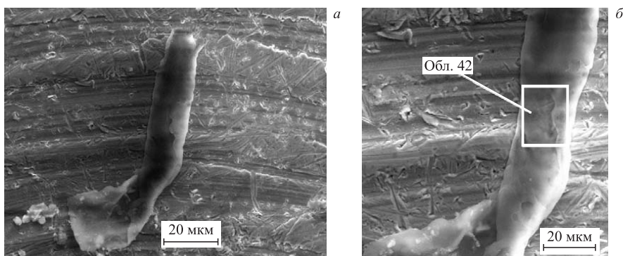
Рис. 7. СЭМ-изображение трубки на поверхности ВО (а) с частью трубки с большим увеличением из выделенной обл. 42, где выполнен РМЗА (б)
