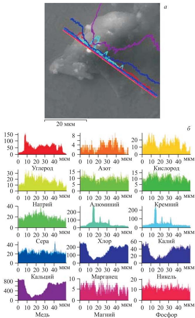
Рис. 25. СЭМ-изображение структуры (а) и концентрации отдельных элементов, полученные сканированием по выделенной полосе (б) на рис. 25, а
