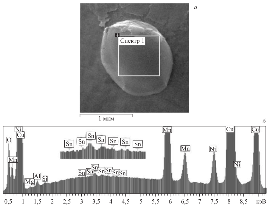
Рис. 28. СЭМ-изображение структуры (а) и спектр ХСРП, полученный в выделенной области (спектр 1) рис. 28, а (б)
