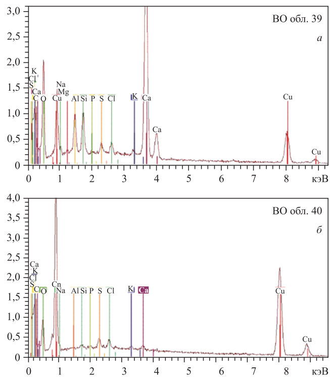
Рис. 5. Спектры РМЗА, измеренные в обл. 39 и обл. 40 на рис. 4, а и б соответственно
