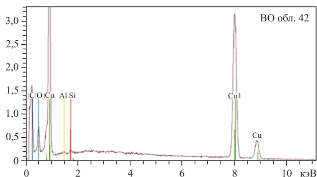
Рис. 8. Спектр РМЗА, измеренный в обл. 42 на рис. 7, б
