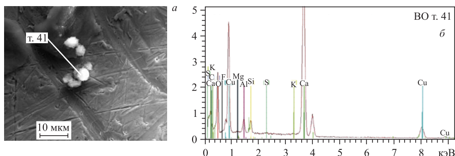
Рис. 6. Изображение скопления частиц на поверхности ВО с выделенной т. 41, где выполнен РМЗА, и спектр РМЗА (б)
