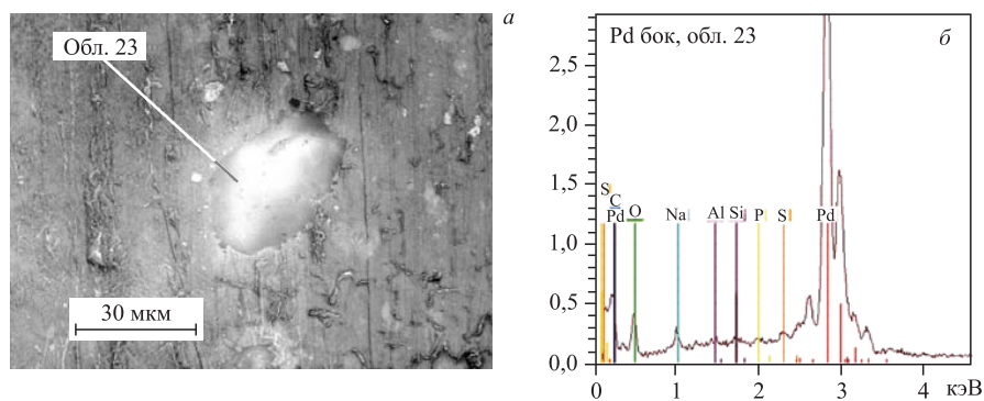
Рис. 14. СЭМ-изображение частицы на поверхности Pd-стержня (а) и РМЗА-спектр, измеренный в обл. 23 (б)
