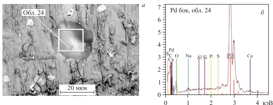
Рис. 15. СЭМ-изображение частицы на поверхности Pd-стержня (а) и спектр РМЗА, измеренный в обл. 24 (б)
