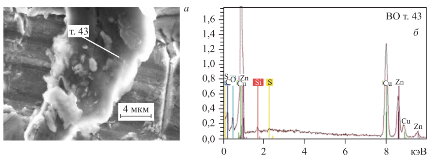
Рис. 9. Изображение частицы на поверхности ВО в выделенной т. 43, где выполнен РМЗА (а), и спектр (б), измеренный в т. 43
