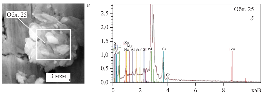
Рис. 16. СЭМ-изображение частицы на поверхности Pd-стержня (а) и спектр РМЗА, измеренный в обл. 25 (б)
