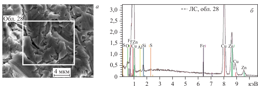
Рис. 32. СЭМ-изображение участка поверхности ЛС ( a ) и спектр РМЗА, проведенного в обл. 28 ( б )
