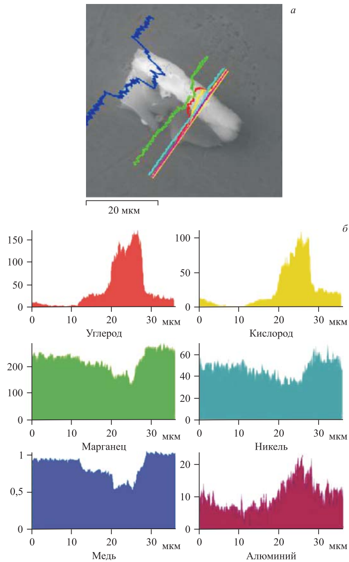
Рис. 24. СЭМ-изображение тонкостенной трубки, край которой не завернулся до конца (а), и концентрации отдельных элементов, полученные сканированием по выделенной на рис. а полосе (б)
