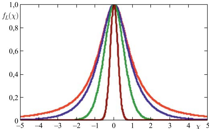
Рис. 2. Функции (1.30) распределения светимости по участку встречи пучков: \alpha = 10; 3; 1; 0,3
