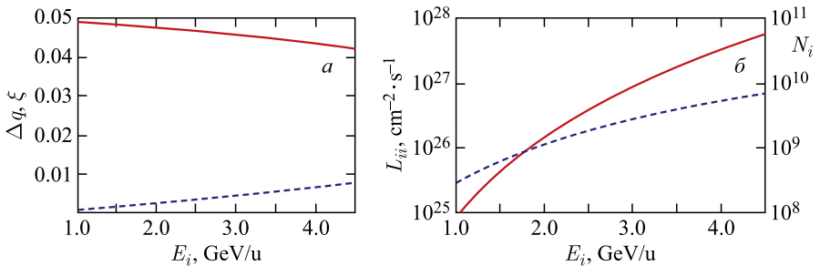
Рис. 4. Зависимость от энергии ионов E_i параметров ионного коллайдера на сгруппированных пучках ^{197}\text{Au}^{79+} ; \Delta Q = 0,05 : a ) параметры Ласлетта \Delta q (сплошная кривая) и эффекта встречи \xi (штриховая); б ) светимость коллайдера L_{ii} (сплошная кривая) и число частиц в сгустке N_i (штриховая)
