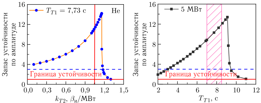
Рис. 8. Запас устойчивости ИБР-4 по амплитуде с твэлами ИБР-2М (He-подслой) в режиме саморегулирования (без АР) при изменении положительного коэффициента передачи МОС k_{T2} (а) и постоянной времени первого компонента МОС T_{T1} (б). Средняя мощность реактора 5 МВт. Красные вертикальные линии — рабочие значения параметров МОС ИБР-2М
