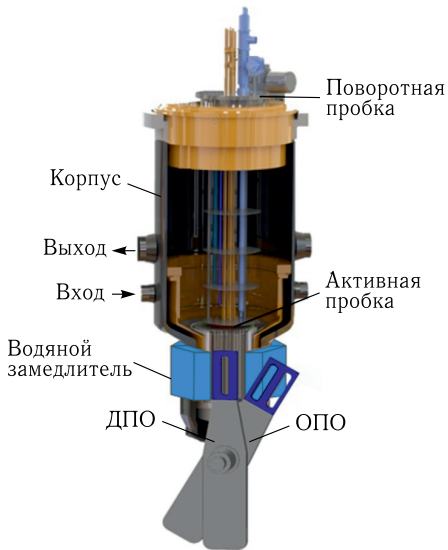
Рис. 3. Корпус ИБР-4 с модулятором реактивности ПО-3
