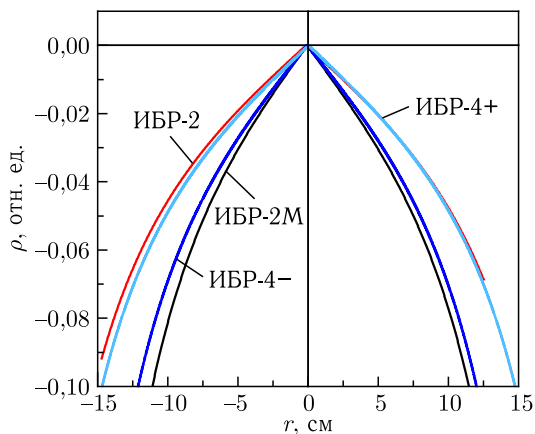
Рис. 12. Аппроксимированная распределенная реактивность в ИБР-2, ИБР-2М и ИБР-4. ИБР-4+ — с выравниванием энерговыделения, ИБР-4- — без выравнивания
