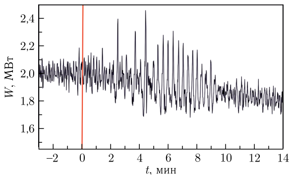
Рис. 4. Появление низкочастотных колебаний в ИБР-2М при штатном снижении средней мощности от 2 до 1,8 МВт в цикле № 9 23-12-2017 г. Красная линия — начало снижения мощности
