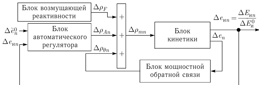
Рис. 5. Блок-схема модели динамики ИБР-4
