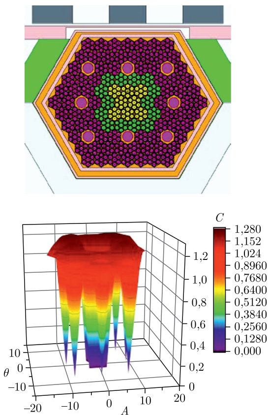
Рис. 11. ИБР-4 с твэлами ИБР-2М и бесчехловыми кассетами: всего 102 ТВС, 86 ТВС с диоксидом плутония, 8 стержней СУЗ с обогащенным бором, 8 ТВС — кассет-имитаторов для компенсации выгорания, 13 ТВС со вставками ВНЖ длиной 6 см в центре каждого твэла
