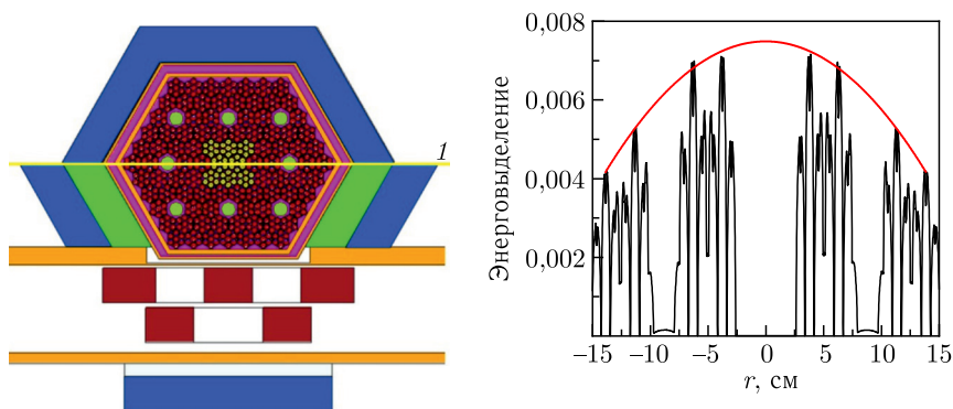
Рис. 9. Распределение энерговыделения по радиусу а. з. ИБР-4 по линии 1
