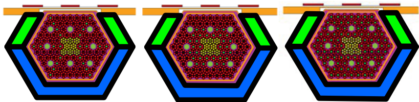
Рис. 15. Способы усиления жесткости некоторых кассет ИБР-4 с целью уменьшения их изгибов к центру а. з. Вольфрамовые стержни введены в центральный твэл
