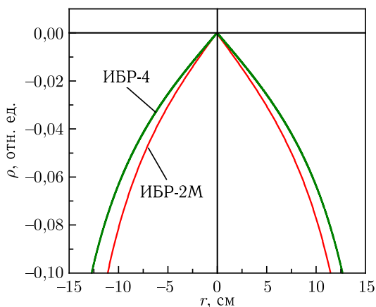
Рис. 10. Аппроксимированная распределенная реактивность в ИБР-2М (красная линия) и в базовой компоновке ИБР-4 (зеленая линия). В среднем градиент распределенной реактивности (или чувствительность) ИБР-4 к смещению топливных кассет только на \sim 15\% меньше, чем в а. з. ИБР-2М
