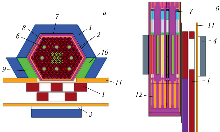
Рис. 2. Расчетная модель ИБР-4: а) поперечный разрез а.з. ИБР-4 с органами СУЗ и имитаторами; б) продольный разрез а.з.: 1 — модулятор реактивности; 2 — двойной корпус; 3 — слой В 4 С; 4 — плоский водяной замедлитель; 6 — органы СУЗ В 4 С (80% 10 В); 7 — слой жидкого натрия; 8 — ТВС; 9 — КО1; 10 — КО2; 11 — корпус модулятора реактивности; 12 — опорная решетка
