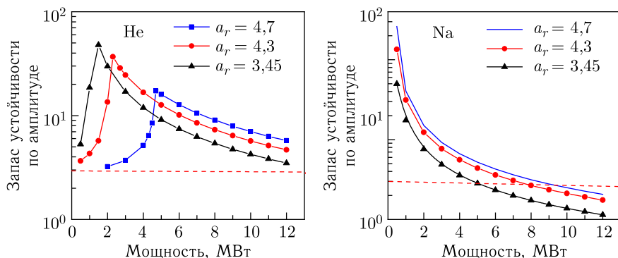
Рис. 13. Запас устойчивости ИБР-4 по амплитуде в режиме саморегулирования для разных твэлов с подслоем He (а) и Na (б) с выравниванием энерговыделения в а. з. в зависимости от мощности реактора; \beta_{и} = 1,85 \cdot 10^{-4}
