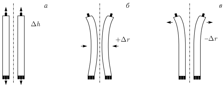
Рис. 6. Схематическое представление действия отдельных компонентов МОС ИБР-2, ИБР-2М и ИБР-4: а — аксиальное расширение топлива; б — изгиб кассет к центру а. з.; в — изгиб кассет к периферии а. з.
