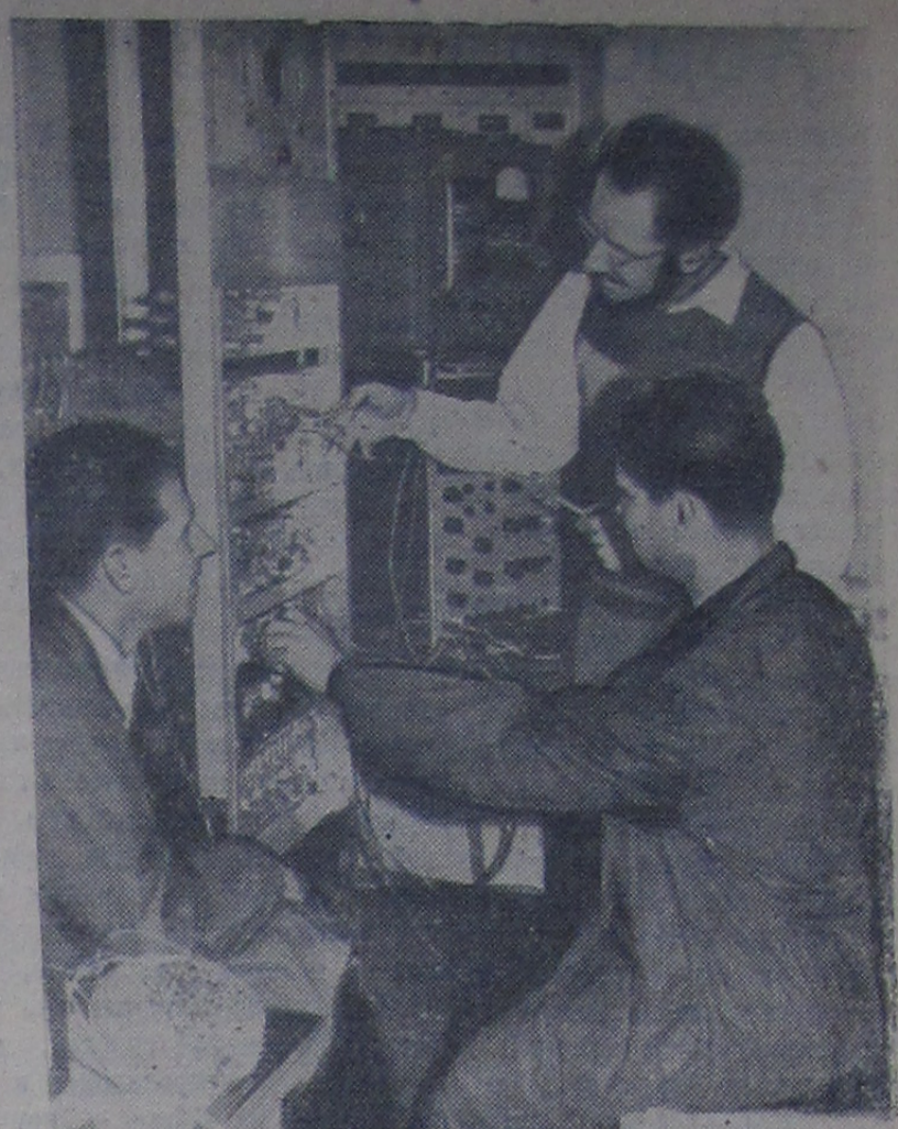
Группа сотрудников Лаборатории ядерных проблем за настройкой узла амплитудного анализатора. На снимке: старший механик А. Фалеев, научный сотрудник А. Сиваев (сидят) и старший инженер из Чехословакии Я. Вавра (стоит).
