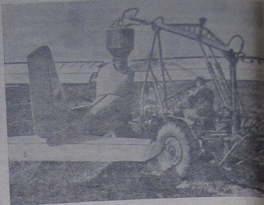
В сельском хозяйстве Чехословацкой Республики широко применяется авиация. На снимке: погрузка минеральных удобрений в бункер самолета «Бригадир». Фото Чехословацкого телеграфного агентства
