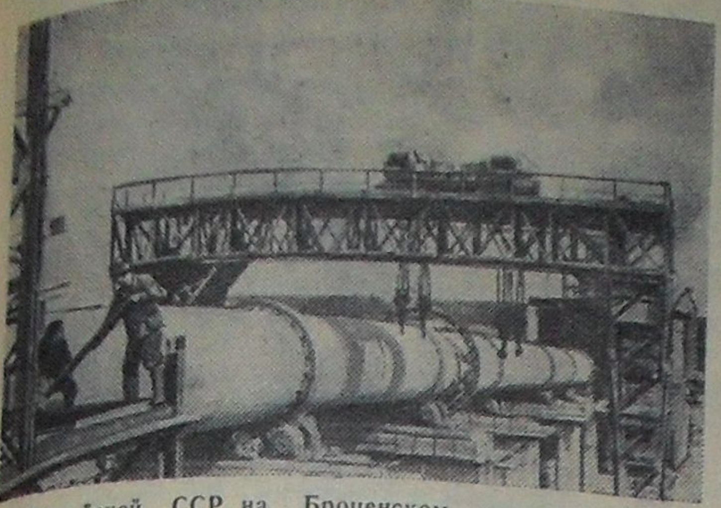
В Латвийской ССР на Броценском цементно-шиферном комбинате сооружается новая технологическая линия. Заключается монтаж 50-метровой вращающейся печи, которая будет производить клинкера значительно больше, чем три действующие. Строятся компрессорная станция, помольное отделение, карьер для добычи глины, шламбассейн. За год новая технологическая линия даст столько цемента, сколько нужно для строительства кварталов на 100 тысяч семей. Строители опережают график: они стремятся завершить работы на месяц раньше намеченного срока.
