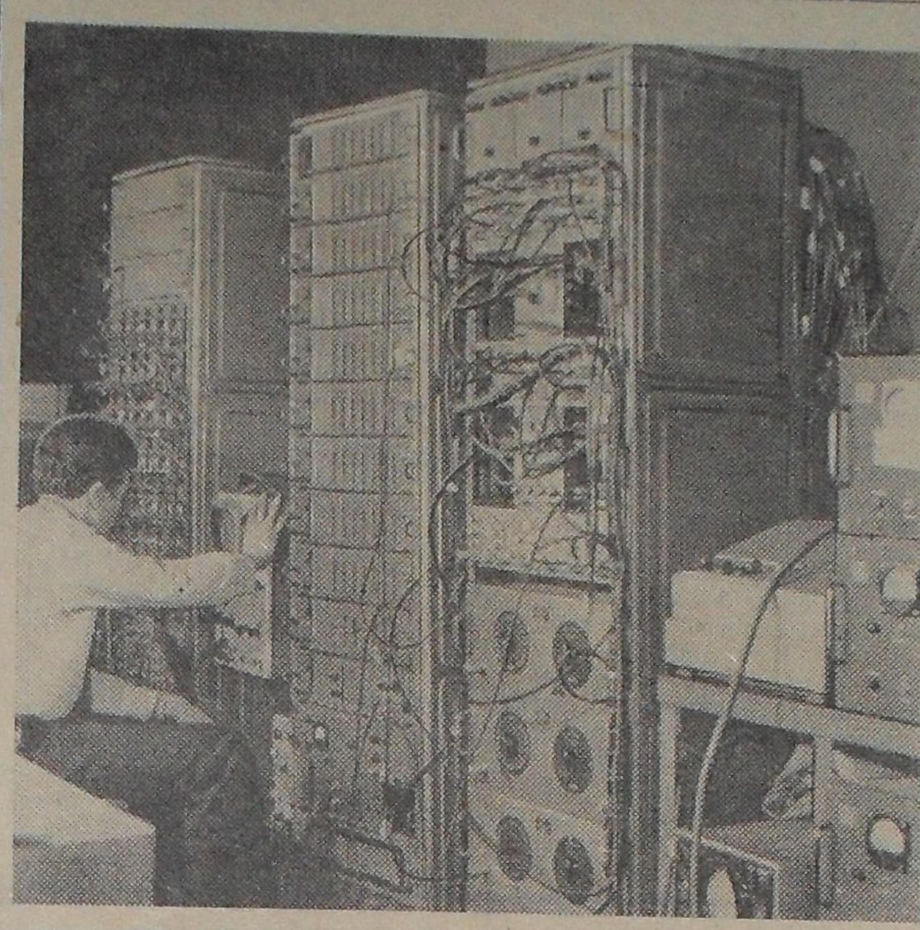
Методика бесфильмовых искровых камер, работающих на линии с ЭВМ, начала развиваться в Лаборатории высоких энергий в 1965 году.
